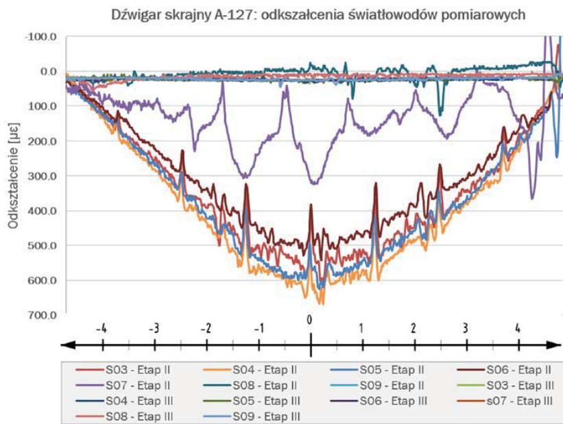
Rys. 10. Dźwigar skrajny A-127: zbiorczy wykres odkształceń w poszczególnych etapach
