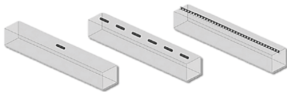
Rys. 1. Graficzna interpretacja pomiaru punktowego, quasi-ciągłego oraz ciągłego (rozłożonego)
